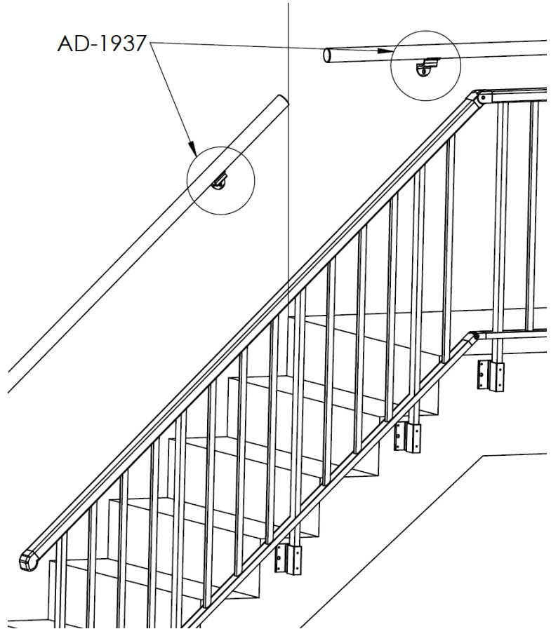
AD-1937 Sujeción pasamanos/pared redondo 50 mm
