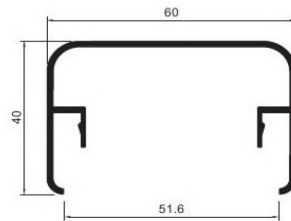
AD-1327 Anclaje Reg Superior Pasamanos 60x40
