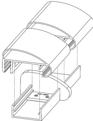
AD-1829 Unión elíptico 85x42.5
