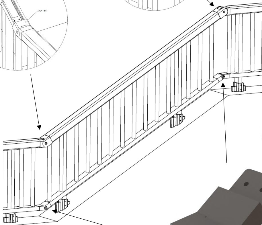
AD-1873 Rótula inferior escalera
