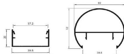
AD-1774 Anclaje telescópico pasamanos red 60
