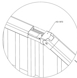
AD-1872 Rótula superior bajada
