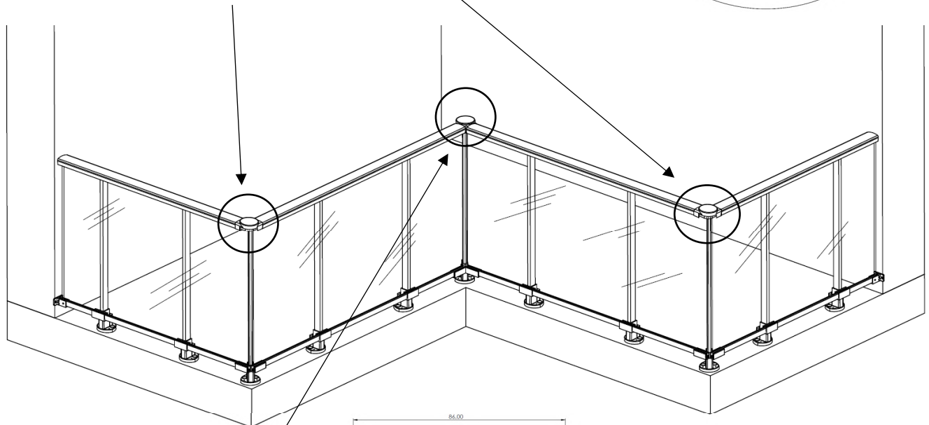
AD-1780 Rótula elíptica con "U" incorporada
