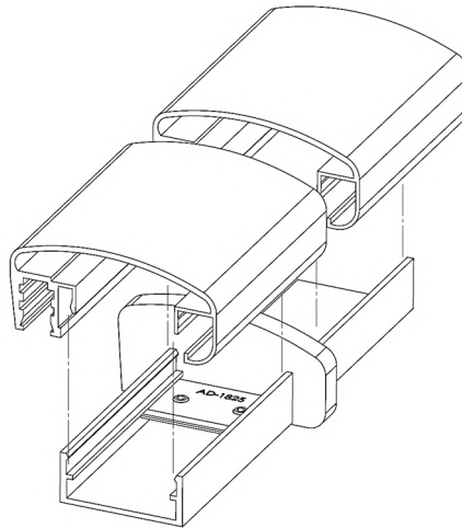
AD-1825 Unión elíptico 86x40
